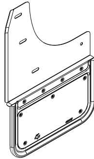
(1) Montaje de aleta, frontal, DS
