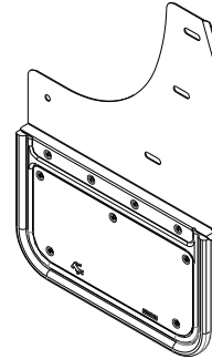
(1) Ensemble de volet, avant côté passager
